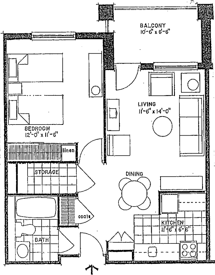
1 bedroom Type B, G 544sf
