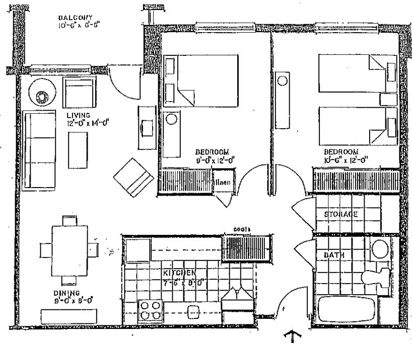
2 bedroom Type A 781 sf
